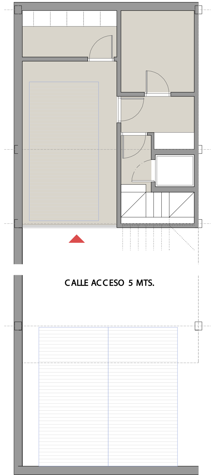
PLANTA SOTANO
