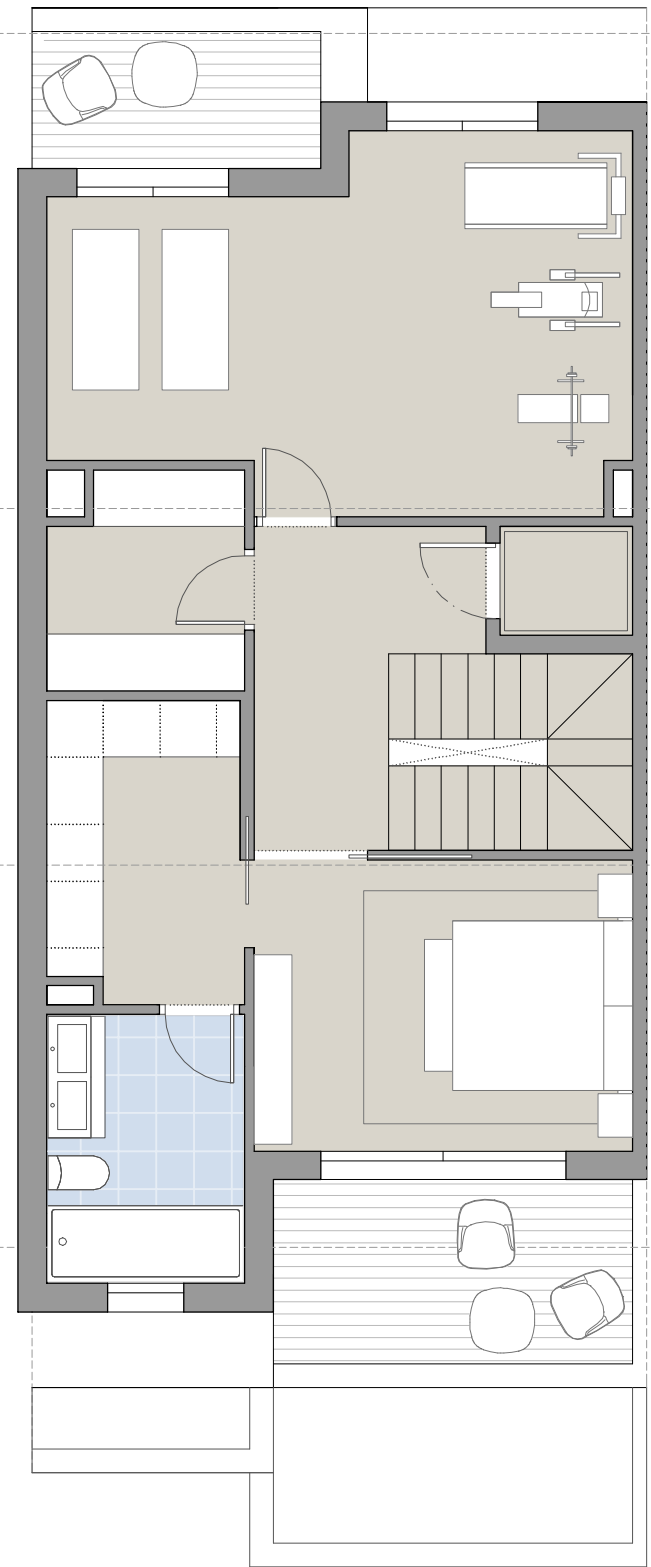
PLANTA SEGUNDA
